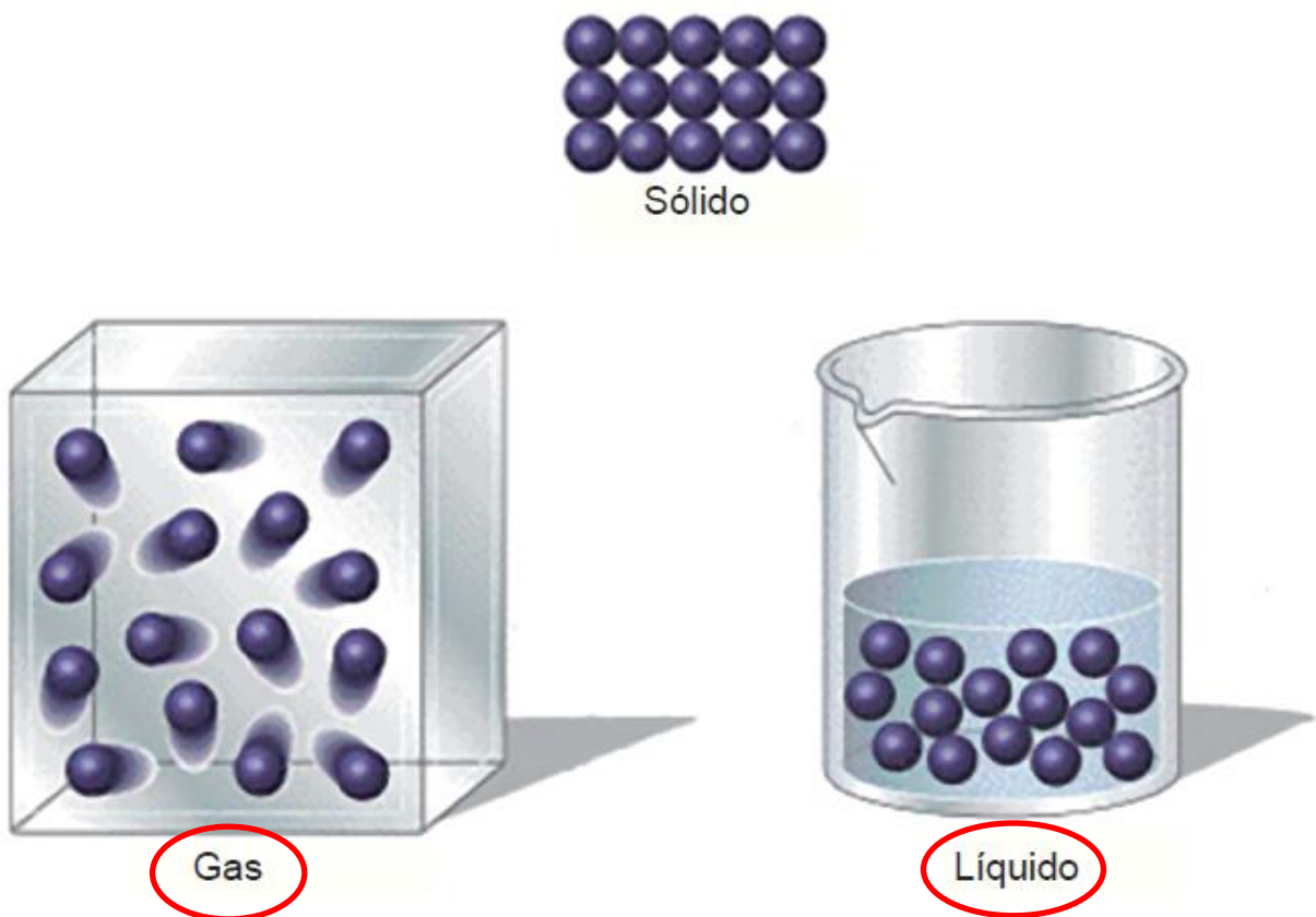
Figura 1.2. Agrupación molecular en función del estado de la materia.
