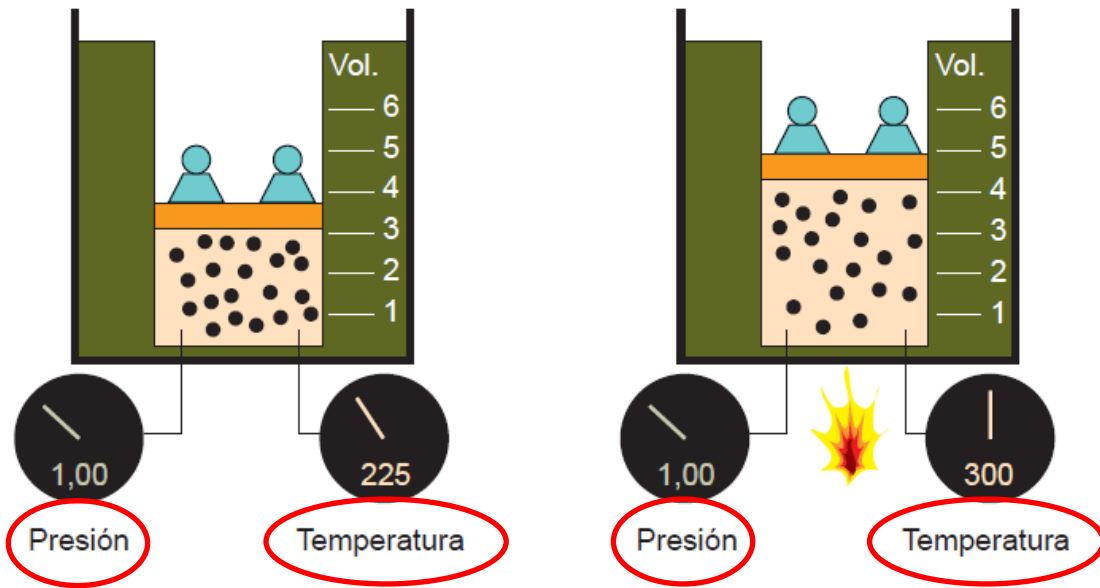
Figura 1.15. Ley de Charles.
