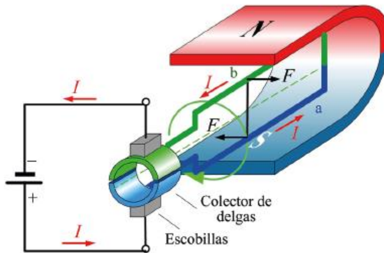
Figura 8.35. Motor de C.C.
