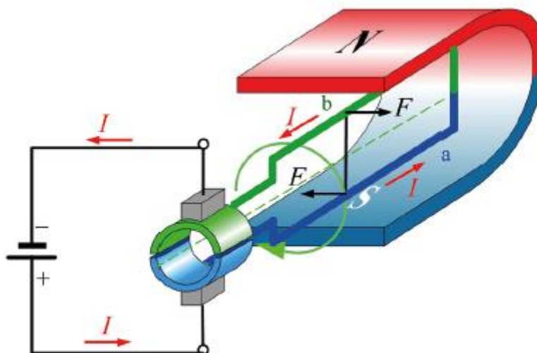
Figura 14.33. Motor de C.C. elemental.
