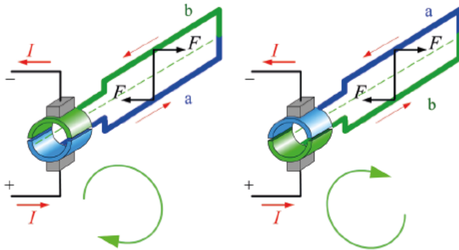
Figura 14.34. Gracias al colector de delgas se consigue que la corriente y la fuerza que aparece en los conductores del rotor sea siempre del mismo sentido.
