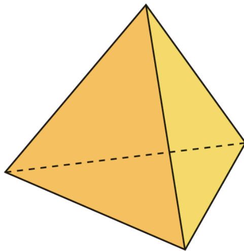
Figura 1.14. Tetraedro o pirámide regular
